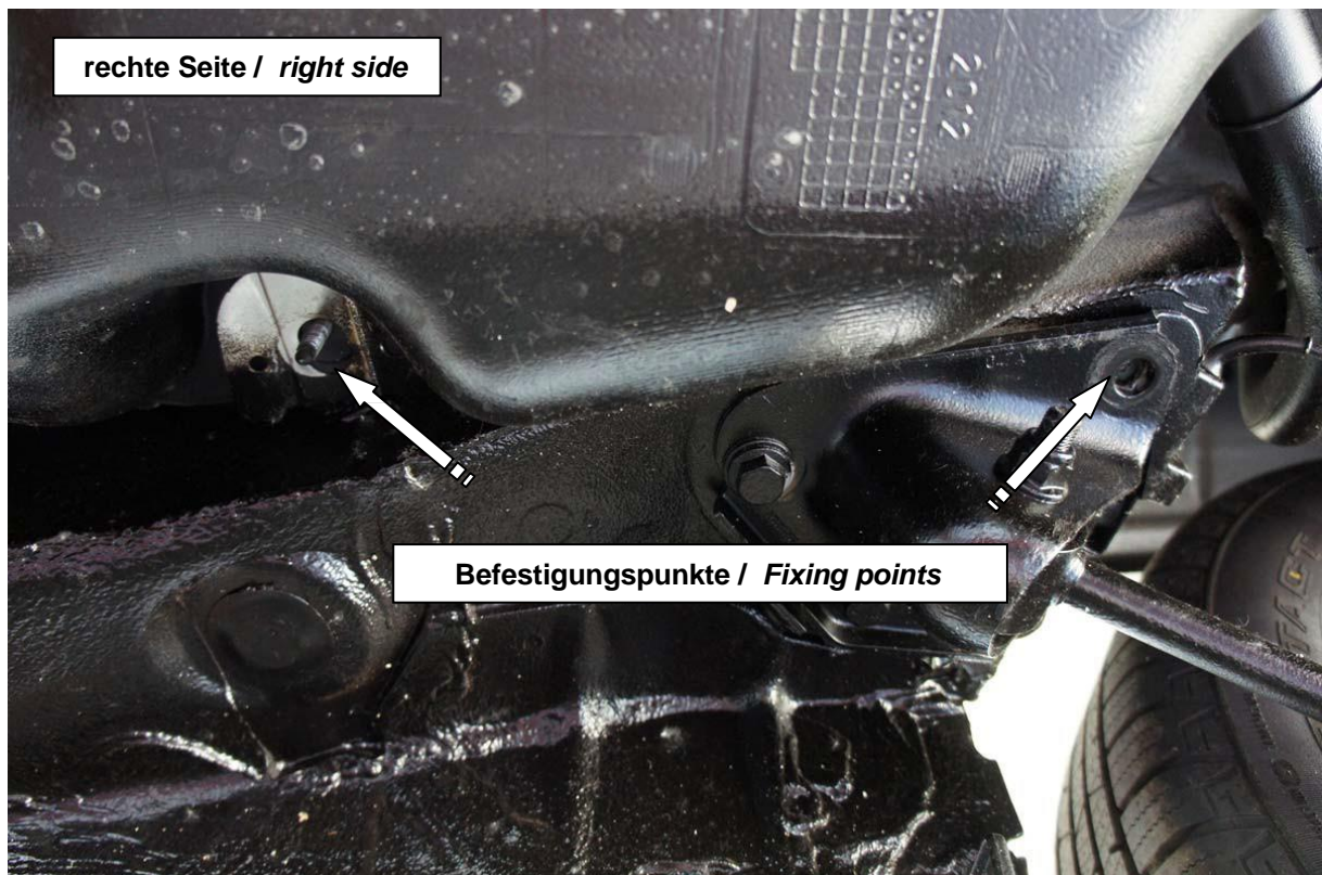
Befestigungspunkte Konsole "B" / Fixing points bracket "B"
