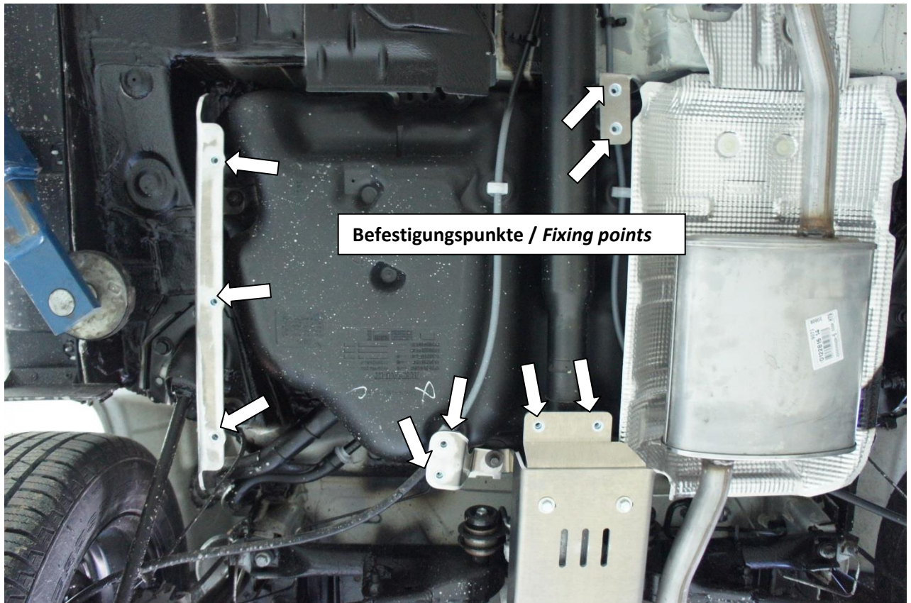
Befestigungspunkte Schutzplatte "A" / Fixing points skid plate "A"
