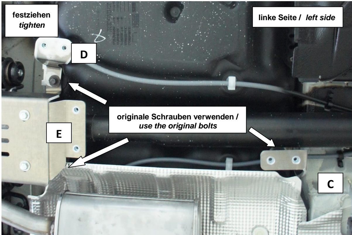
Konsole "C", "D", "E" anbringen / Attach bracket "C", "D", "E"
