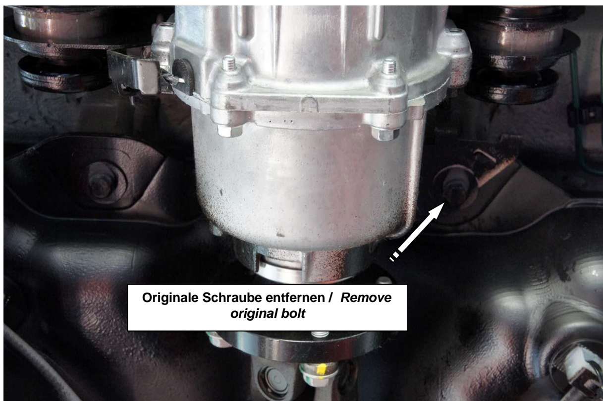
Originale Schrauben entfernen / remove the original bolts
