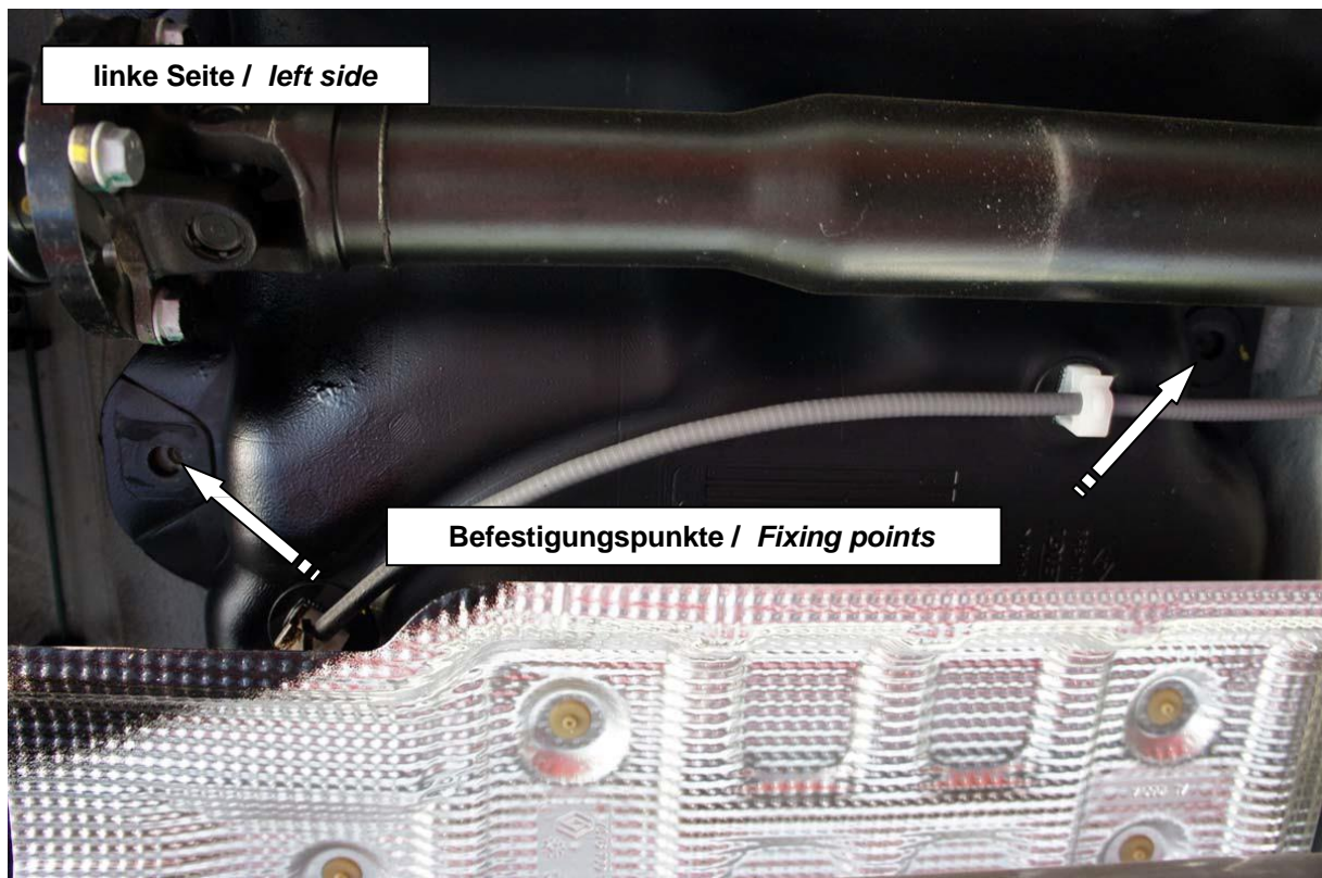
Befestigungspunkte Konsole "C" / Fixing points bracket "C"
